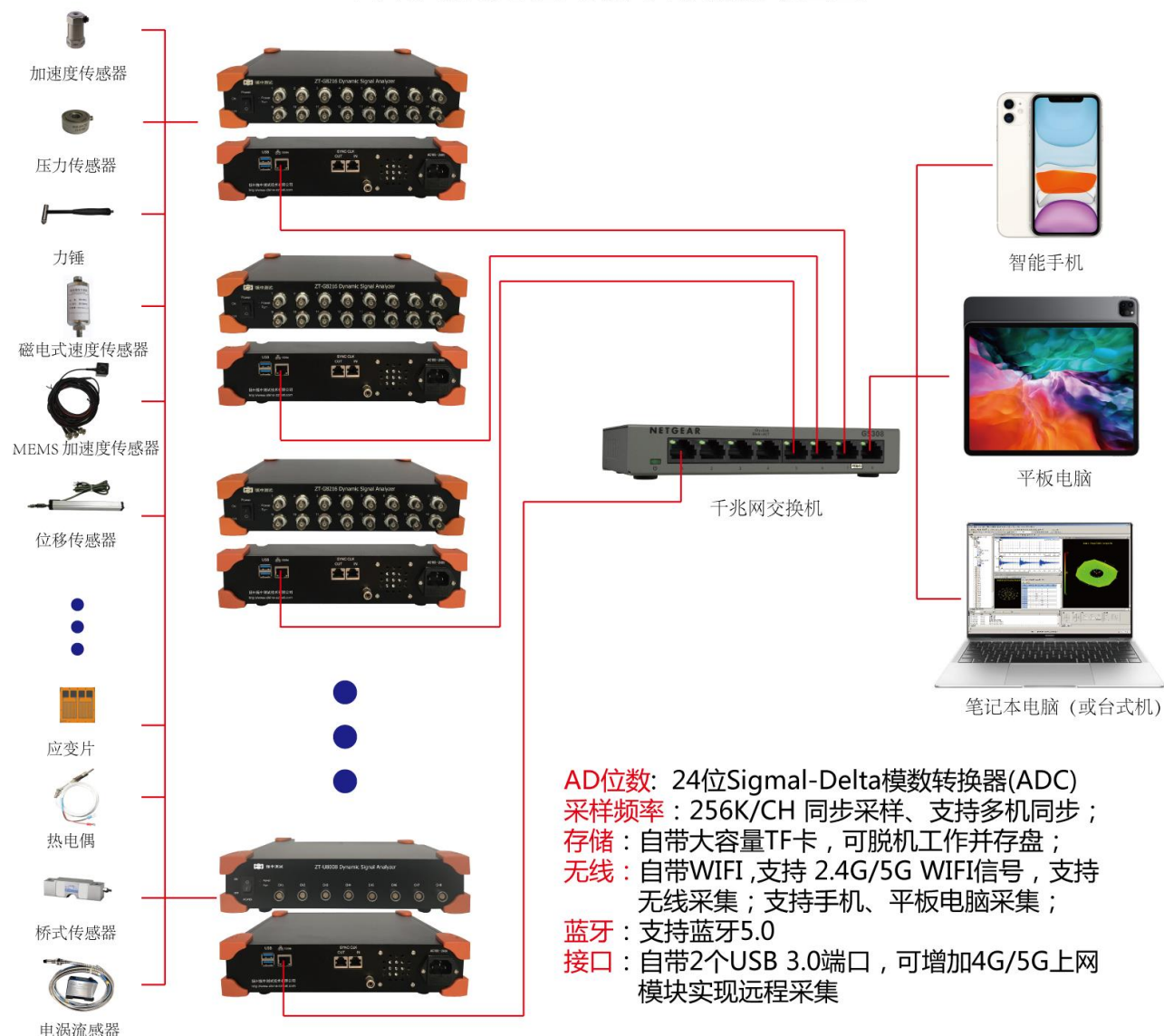
千兆网系列信号分析仪测试框图
